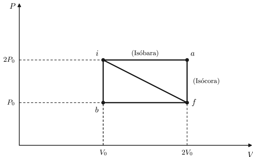
Figura 3.3. El trabajo depende de la trayectoria.
