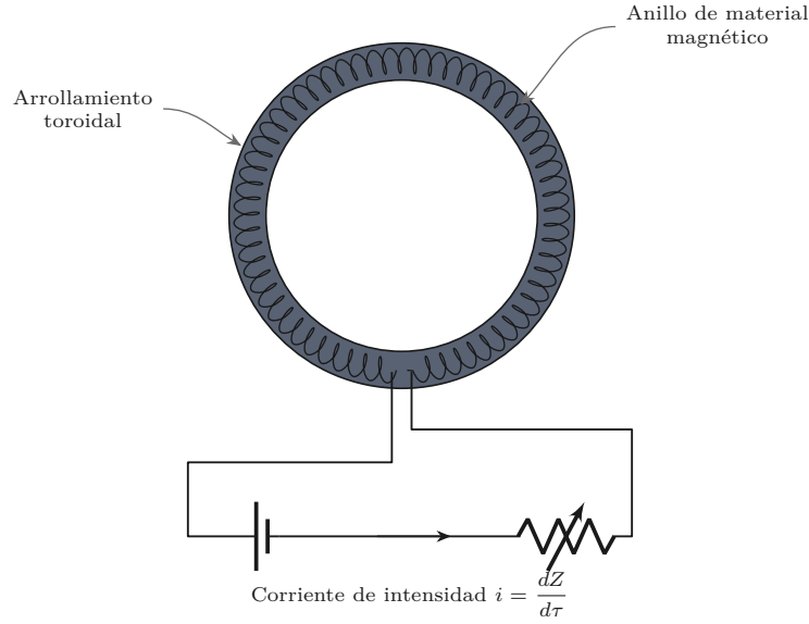
Figura 3.7. Variación de la imanación de un sólido magnético.
