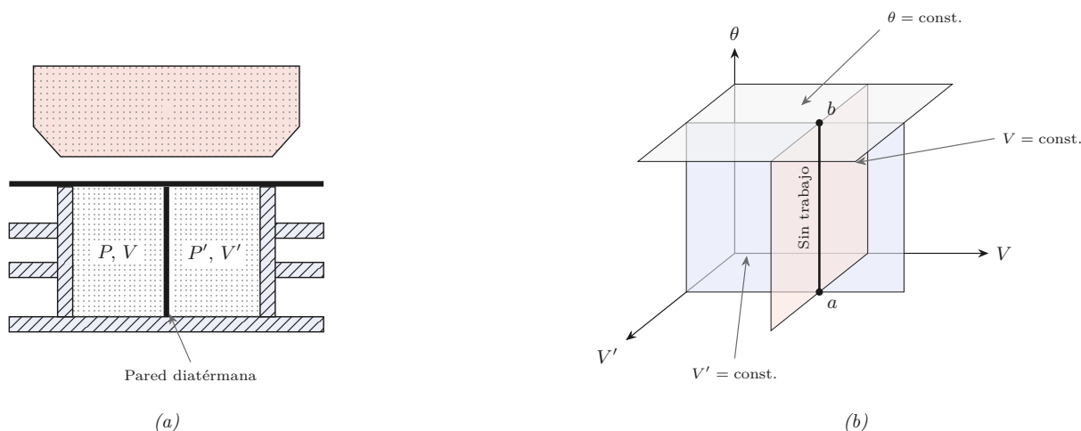
Figura 3.8. (a) Sistema compuesto cuyas coordenadas son P, V, P', V' y \theta . (b) Gráfica de las coordenadas independientes \theta, V y V' .
