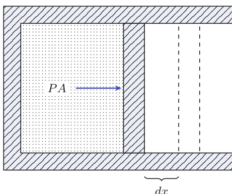
Figura 3.1. Contracción cuasi-estática de un sistema hidrostático.
