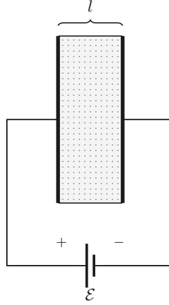
Figura 3.6. Variación de la polarización de un sólido dieléctrico.
