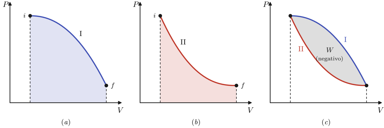
Figura 3.2. Diagrama PV. (a) Curva I, expansión; (b) Curva II, compresión; (c) Curvas I y II, juntas constituyen un ciclo.
