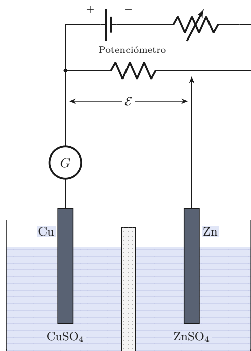
Figura 3.5. Transferencia de carga, aproximadamente cuasi-estática, en una pila reversible.
