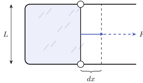
Figura 3.4. Lámina superficial extendida sobre un armazón de alambre.
