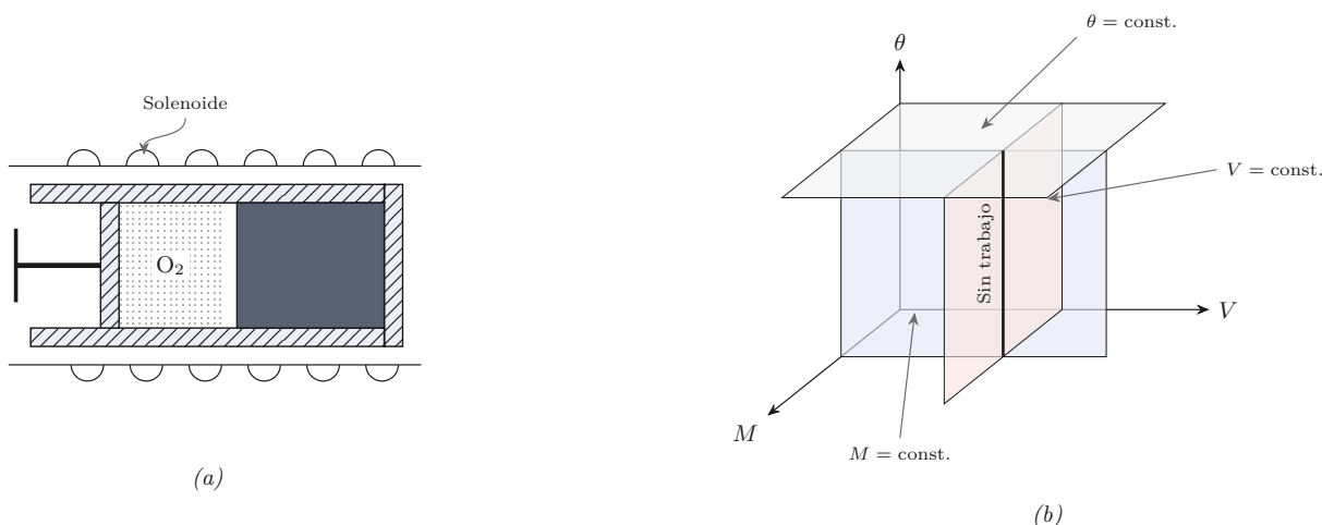
Figura 3.9. (a) Sistema compuesto cuyas coordenadas son P, V, M y \theta . (b) Gráfica de las coordenadas independientes \theta, V y M .
